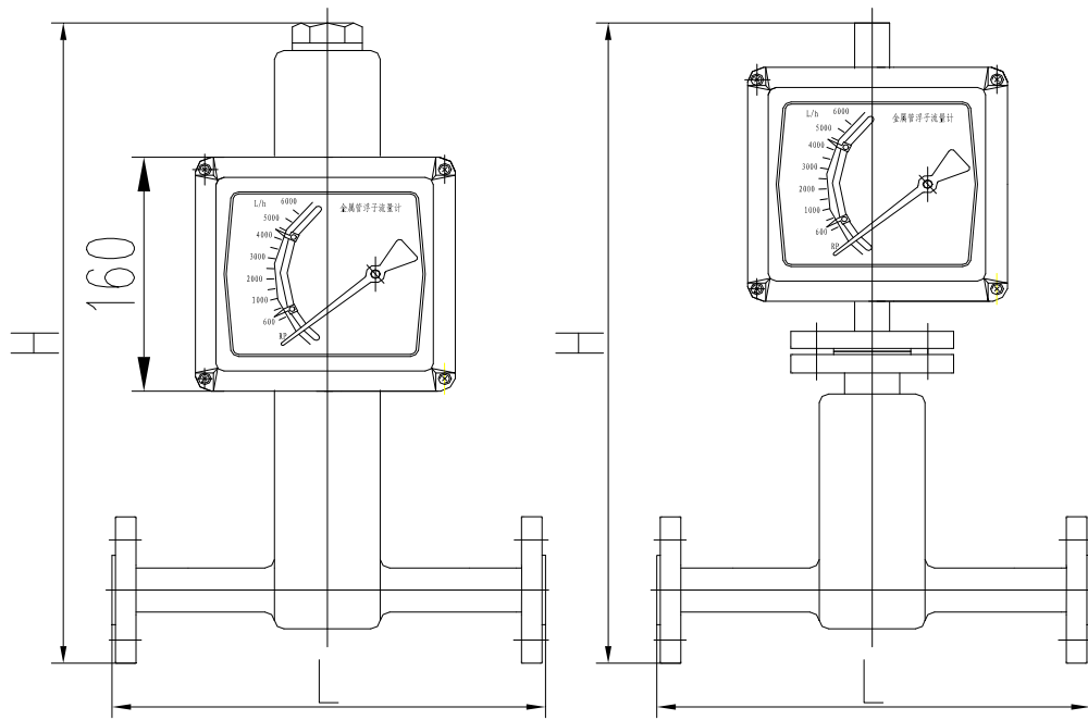
水平安装 (DN15~25)
