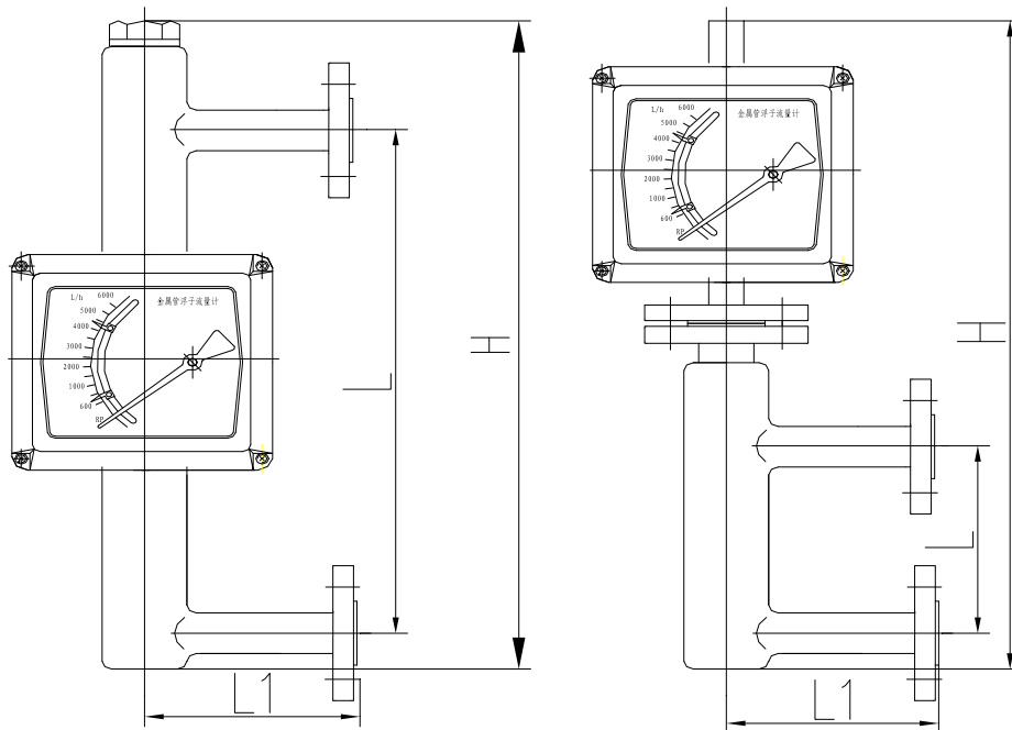
侧进侧出 (DN15~25)
