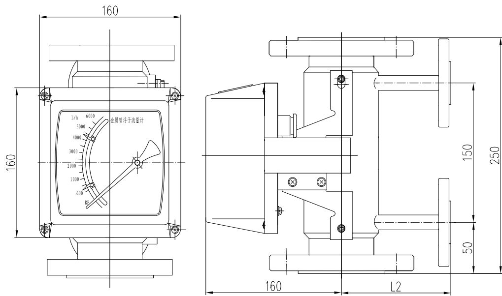
垂直(夹套)安装
